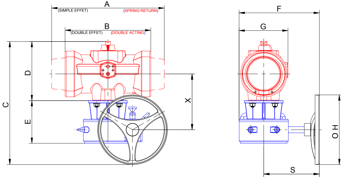
DIMENSIONS ACTIONNEUR + REDUCTEUR DIMENSIONS ACTUATOR + GEARBOX
