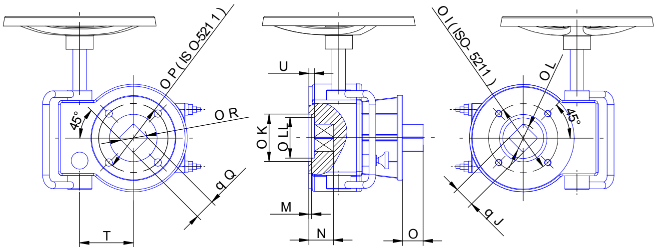
DIMENSIONS REDUCTEUR GEARBOX DIMENSIONS
